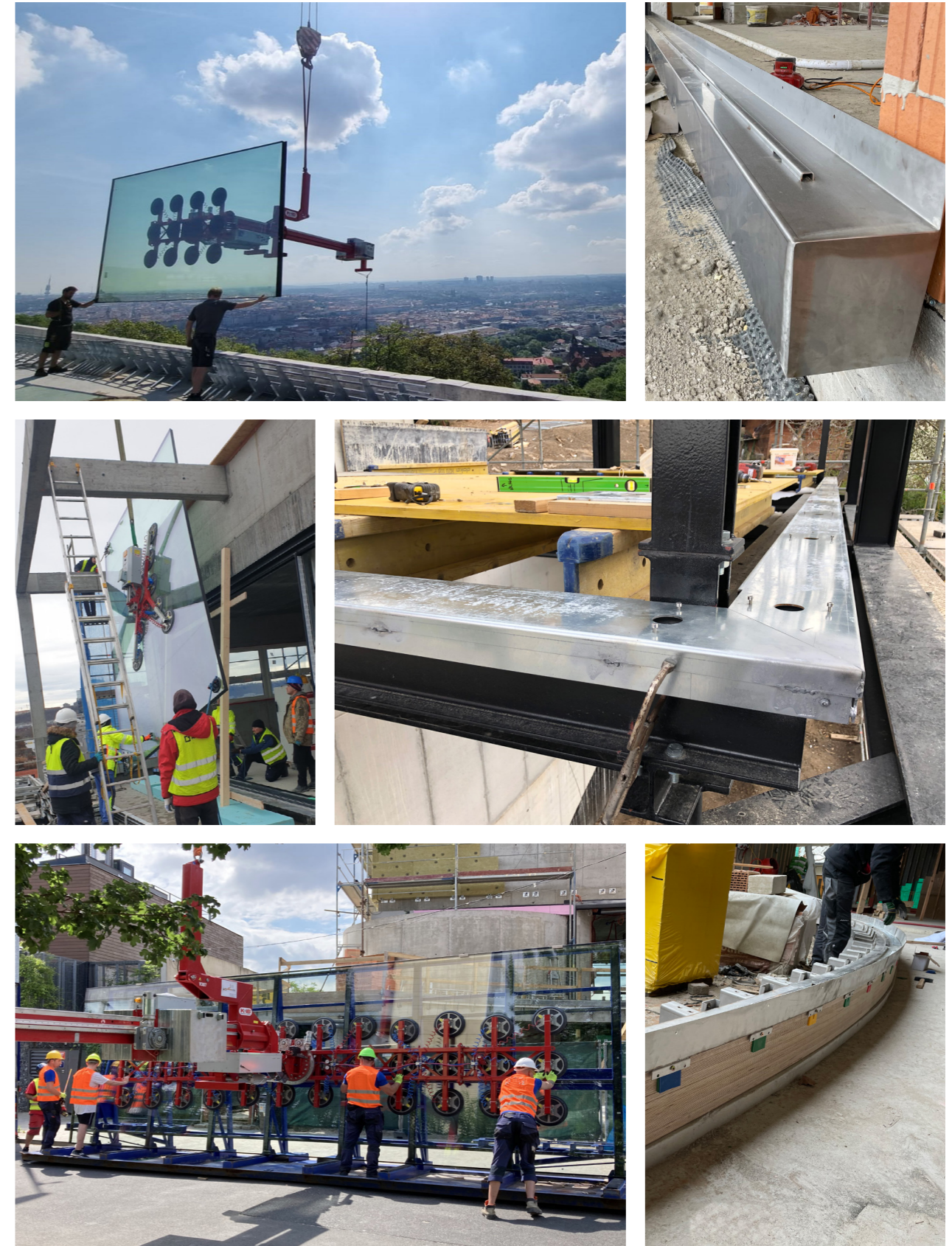
Ukázky práce společnosti Arnold 1990 při instalaci systému air-lux. Manipulace s mnohatunovými břemeny v náročných podmínkách při dodržení milimetrové přesnosti vyžaduje zkušenosti a mnoho šikovných rukou.
